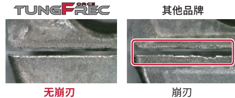
在加工时间相同的情况下切削刃磨损对比
