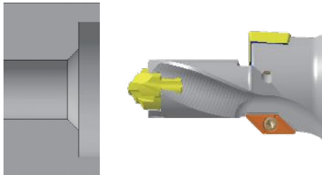
钻孔 + 扩孔 + 倒角
