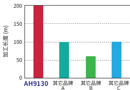
■ 加工碳钢的刀具寿命 (S55C / C55)
