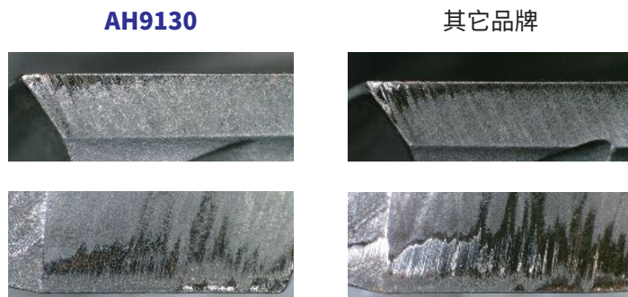
■ 加工 100 m 后刃口磨损情况
