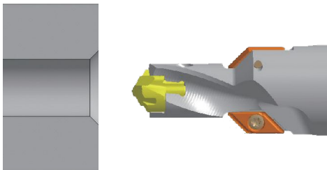
钻孔 + 倒角
