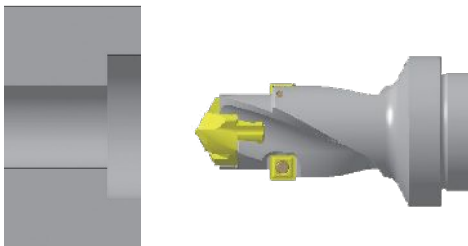
钻孔 + 扩孔
