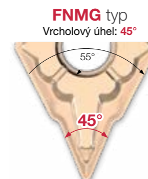
FNMG1104 destička s úhlem špičky 45°: dobrá alternativa k destičkám DNMG s úhlem špičky 55°
