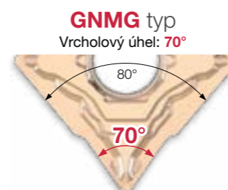
GNMG0904 destička s úhlem špičky 70°: dobrá alternativa k destičkám CNMG s úhlem špičky 80°
