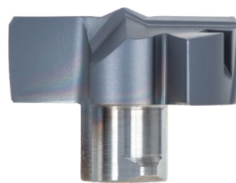
DMF ø6 - ø25.9 mm Arêtes de coupe à 180° pour le lamage et la réalisation de trous à fond plat
