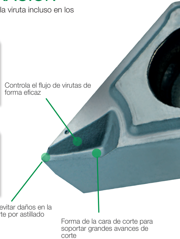
CCGT
