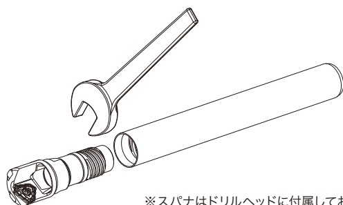
※スパナはドリルヘッドに付属していません。
