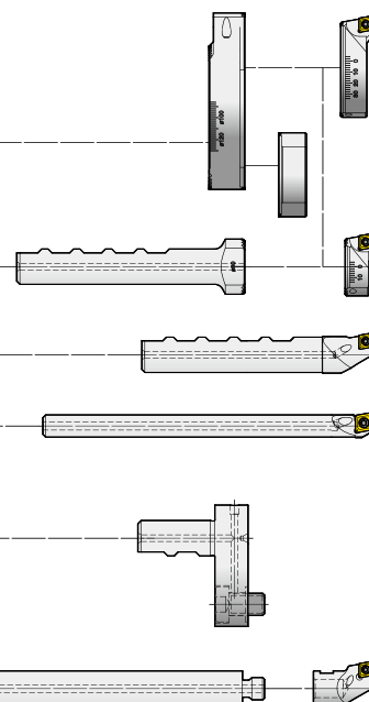
ボーリングホルダ
