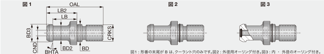
図1：形番の末尾がBは、クーラント穴のみです。図2：外径用オーリング付き。図3：内・外径のオーリング付き。
