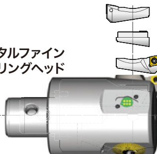
ファインボーリングヘッド 210
