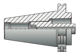
SK: DIN69871
