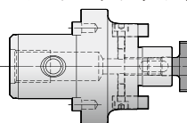
NCドリルチャック
