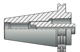
SK: DIN69871
