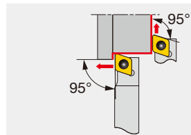
Cutting edge style L2
