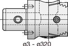
デジタルファインヘッド 206
