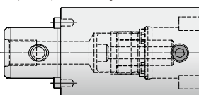
エクステンション
