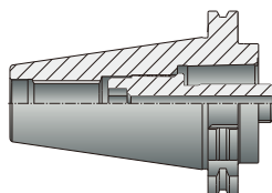
SK: DIN69871
