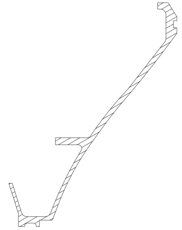
Section cut A-A Scale: 1:2
