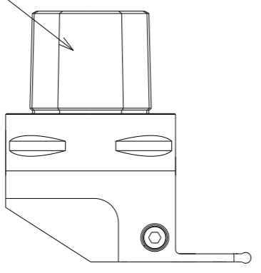
Special Tool TungCut AH8000
