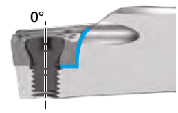
Classique (CCMT060204...pour barre d'alésage)
