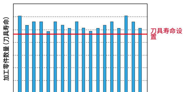
■ DrillMeister 刀具寿命波动
