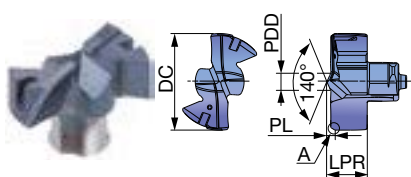
DRILLMEISTER DMF060 - DMF259
