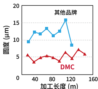
圆度
