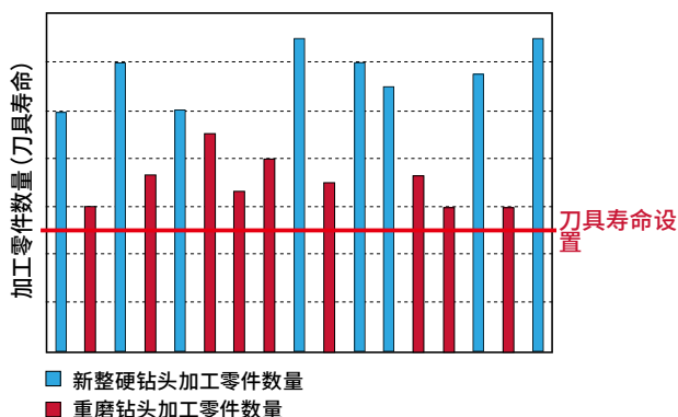
■ 整硬钻头刀具寿命波动
