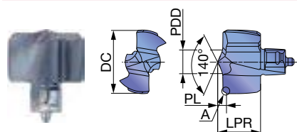
ADDMEISTERDRILL DMF040 - DMF059
