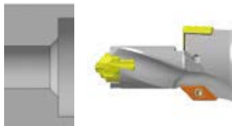
钻孔 + 扩孔 + 倒角
