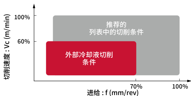
使用外部冷却液时的最佳切削参数设置
