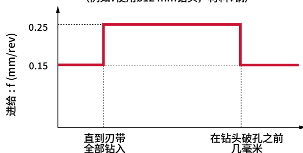
钻削 12×D 通孔时的进给量设置 (例如: 使用 Ø12 mm 钻头, 材料: 钢)
