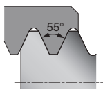
惠氏, 平行管螺纹
