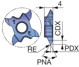
图示为右手型 (R)
