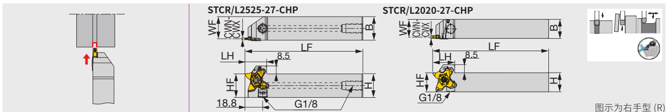
图示为右手型 (R)
