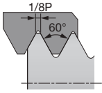
UNJ ( 航空航天工业 )
