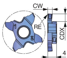
图示为右手型 (R)
