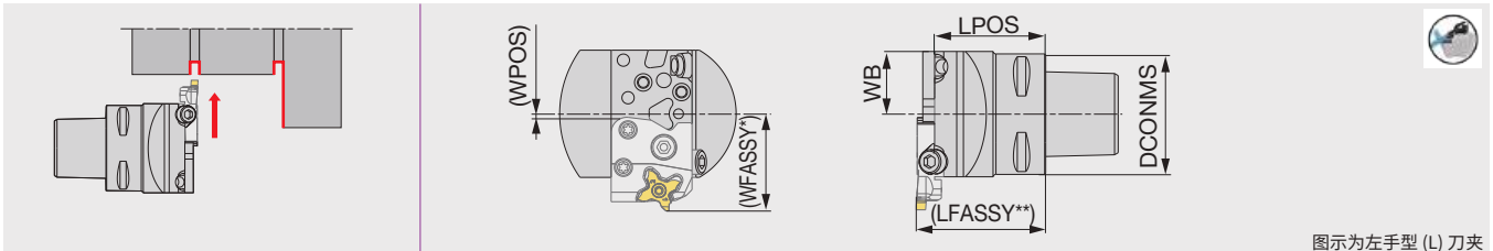
图示为左手型 (L) 刀夹
