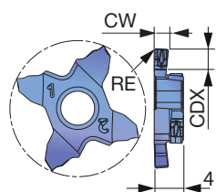
图示为右手型 (R)
