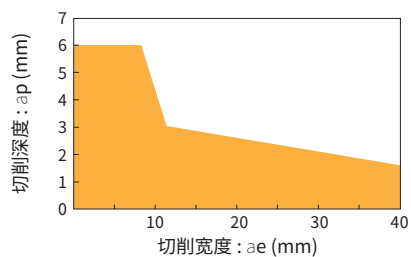
切削深度与切削宽度的关系 (最大切削深度为 \phi 18 mm)
