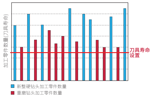
■ 整硬钻头刀具寿命波动
